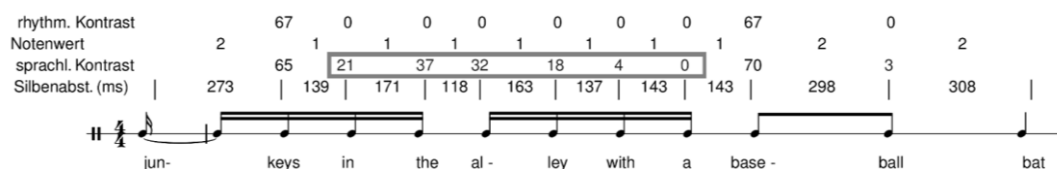
Abb. 1: Oben stehen die transkribierten Notenwerte einer Passage aus der ersten Zeile von Melle Mel (Grandmaster Flash and the Furious Five, »The Message«, 1982, ca. bei Minute 1:15). Über den Notenwerten steht der allein auf ihnen basierende rhythmische Kontrast nach Daniel und Patel (2013). Achtel und 16tel stehen im Verhältnis 2:1, was einem Kontrast von 67% entspricht. Gleich lange Tondauern haben den Kontrast 0.
